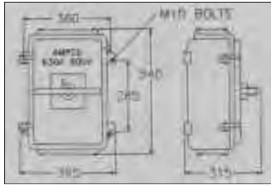
DIMENSIONS: INmm
