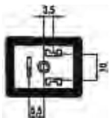
DIN Version
